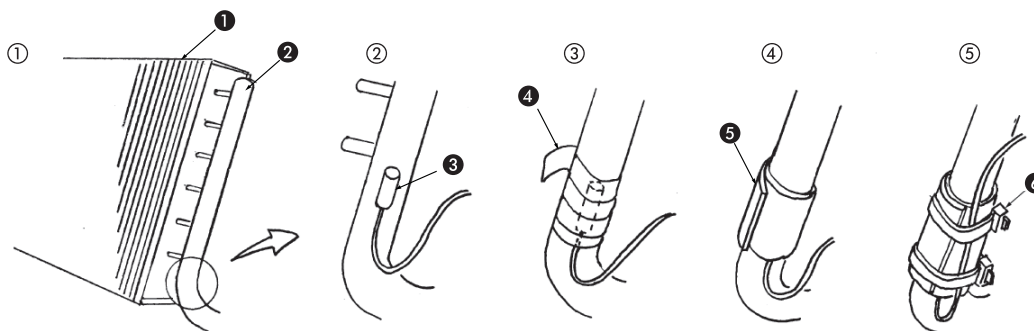
❶ Теплообменник приточной установки ❷ Фреоновый провод (газ) ❸ Датчик температуры ❹ Алюминиевая лента (не входит в комплект поставки) ❺ Теплоизоляция ❻ Кабельная стяжка
