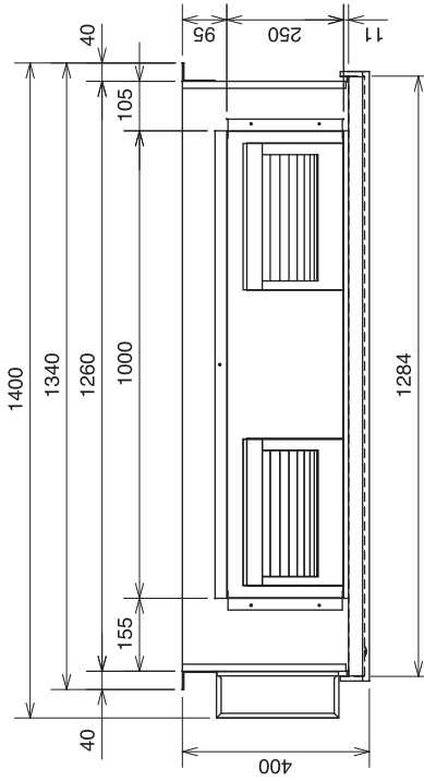
Вид спереди
