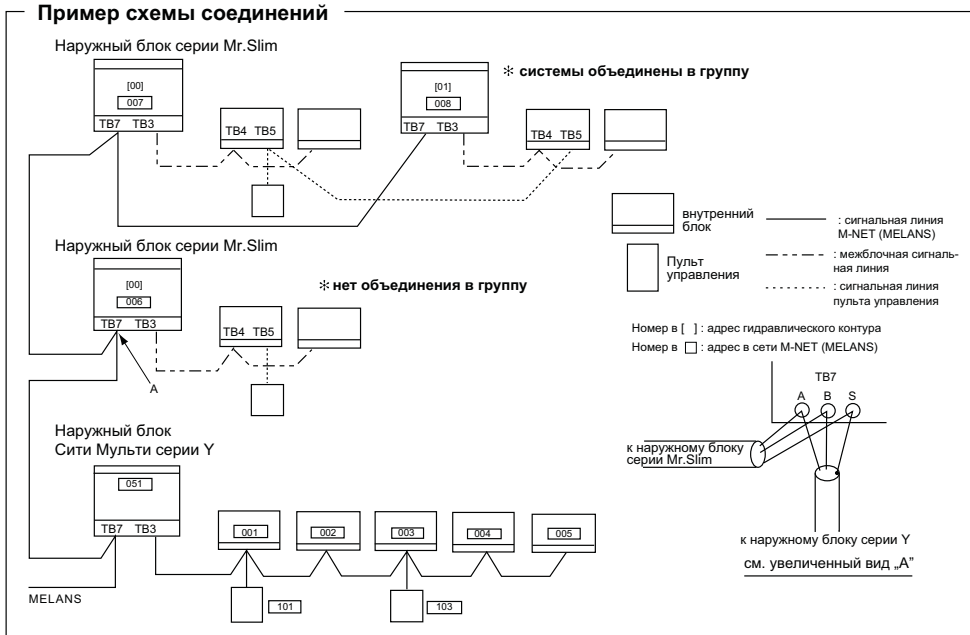
MELANS к клемме TB7 наружного блока
